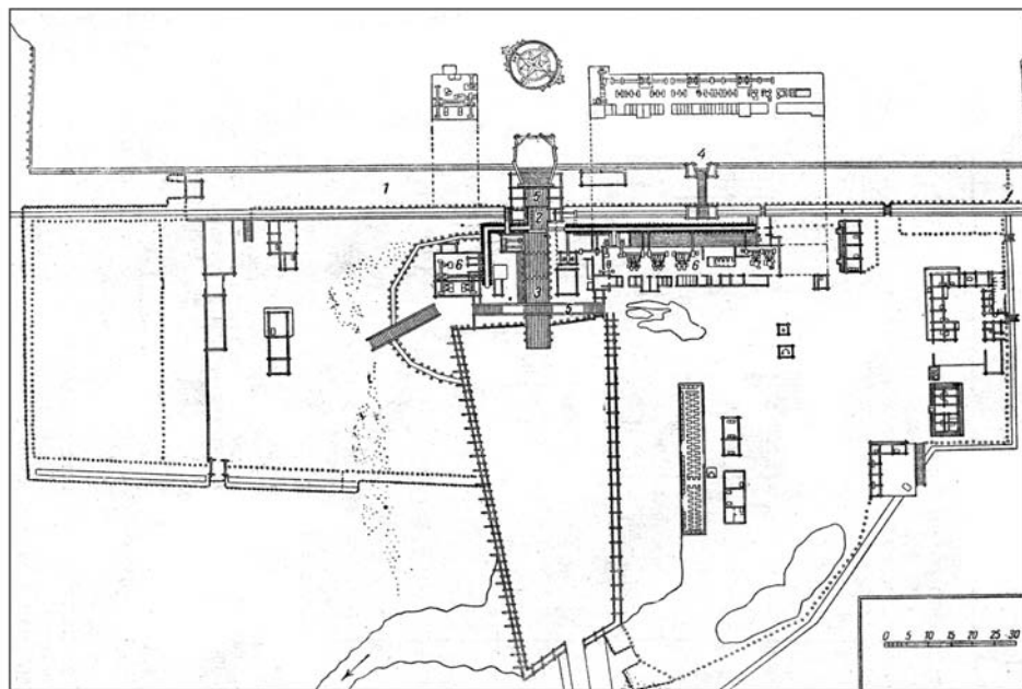
Рис. 12. Барнаульский завод в 1751 г., по чертежу, засвидетельствованному И. И. Ползуновым. 1—плотина; 2—водоспуск; 3—сливной мост; 4—ларевой прорез; 5—мосты через водоспуск и сливной мост; 6—сереброплавильный завод (ЦГАНХ, Л.).
