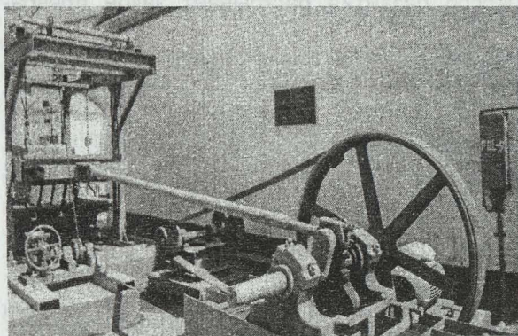
Машина по распиловке камня
